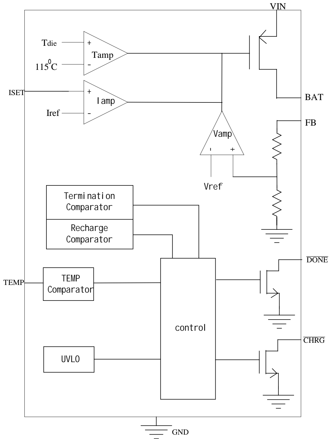
图 3 功能框图
