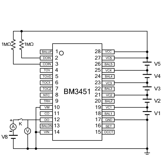
测试电路 7
