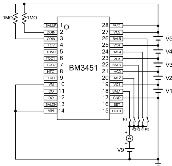
测试电路 8
